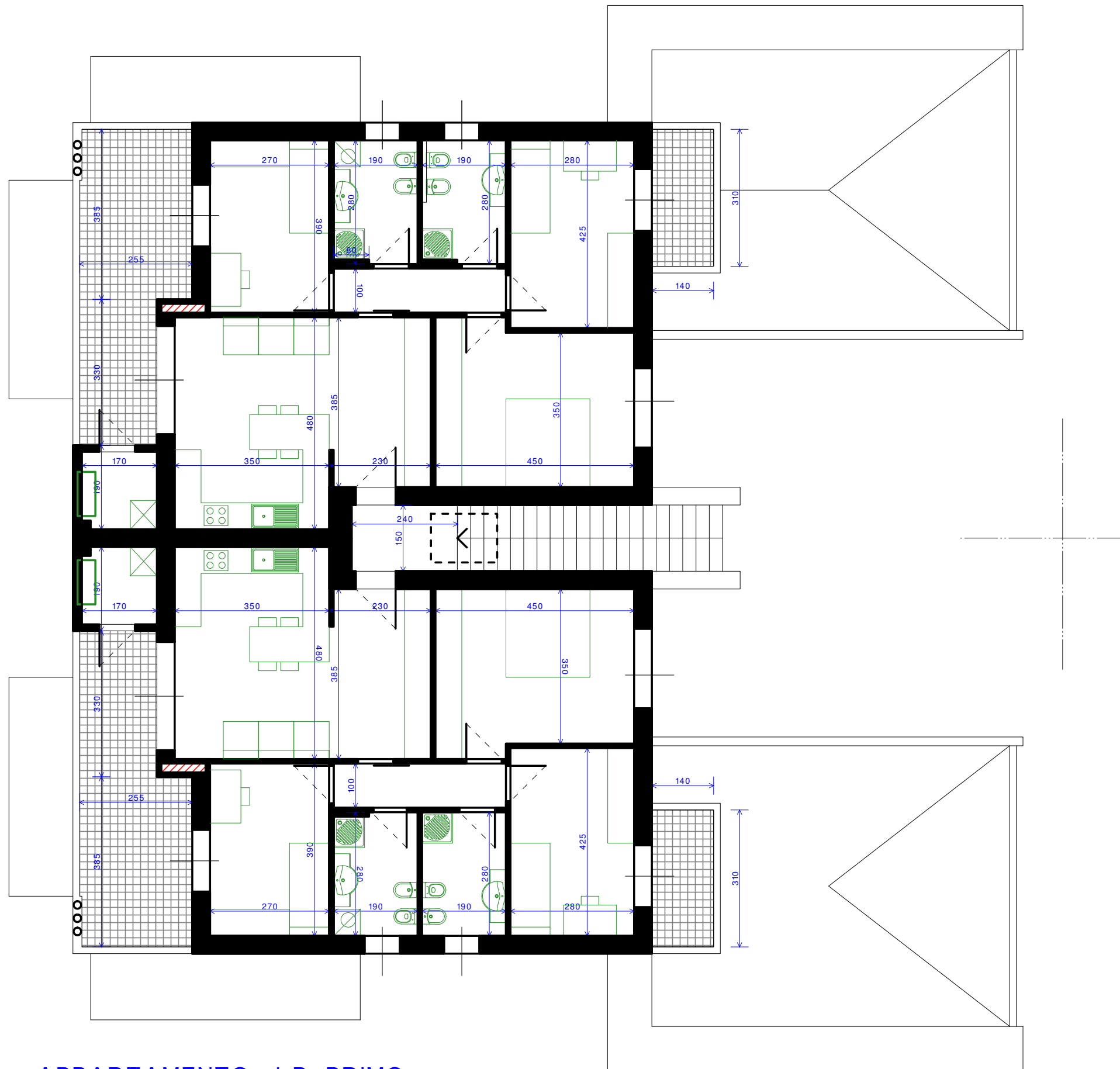
APPARTAMENTO al P. PRIMO TIPO "C" (VARIANTE TRICAMERE)
