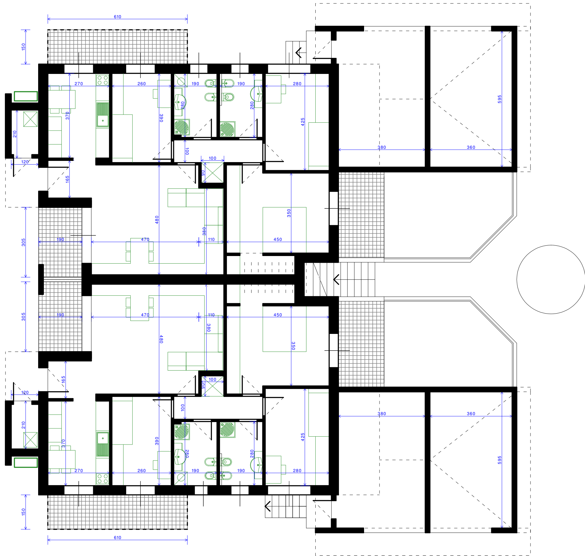
APPARTAMENTO al P. TERRA TIPO "B"
