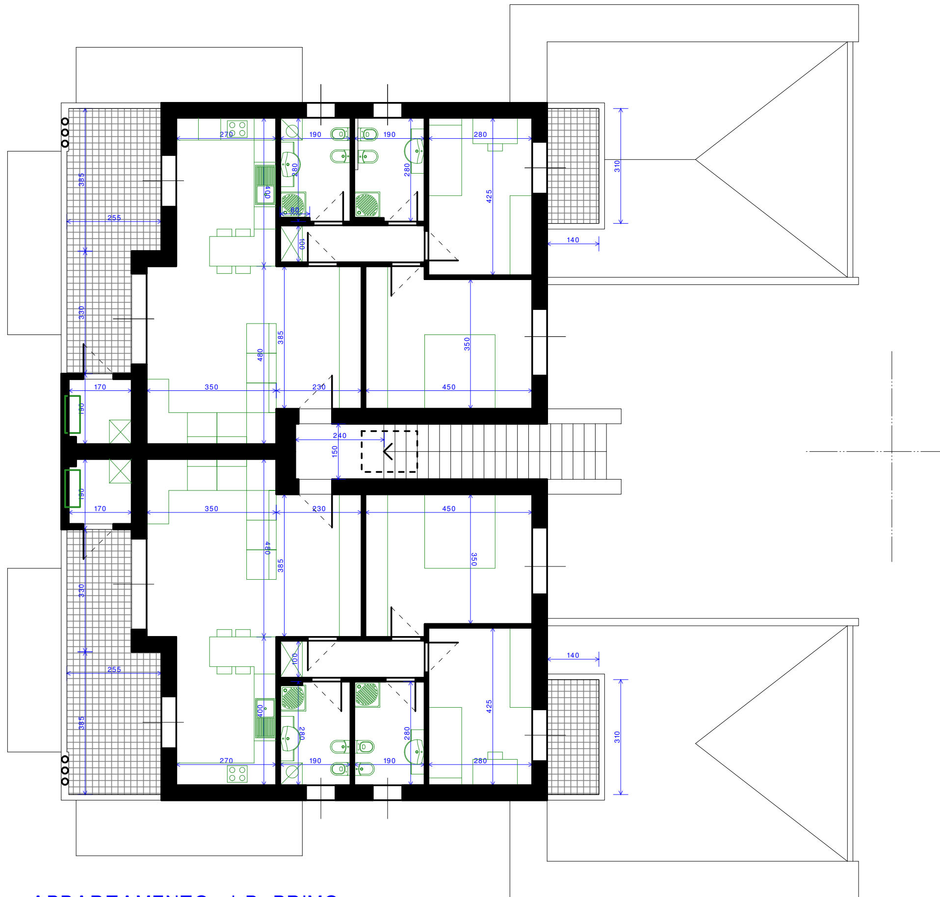
APPARTAMENTO al P. PRIMO TIPO "C"
